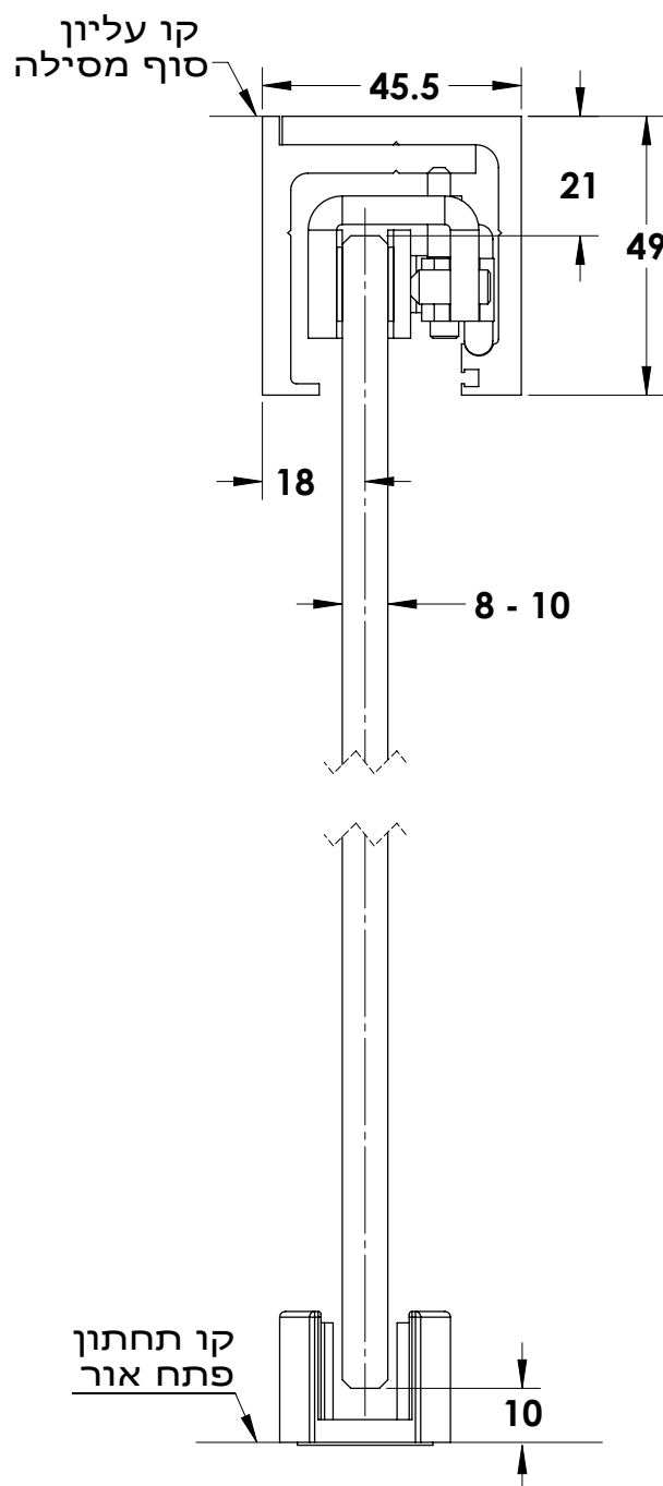
מסילה בחיבור צד
