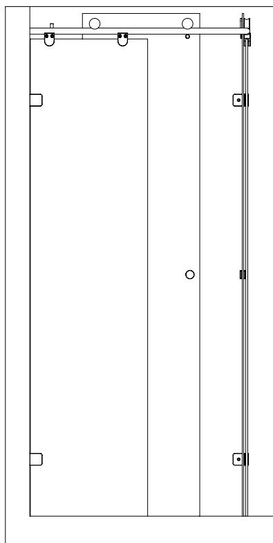
חזית
