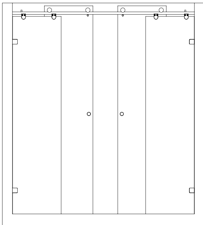
חזית
