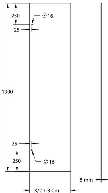
חזית
