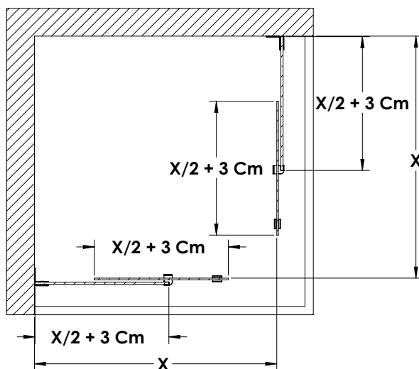
תכנית
