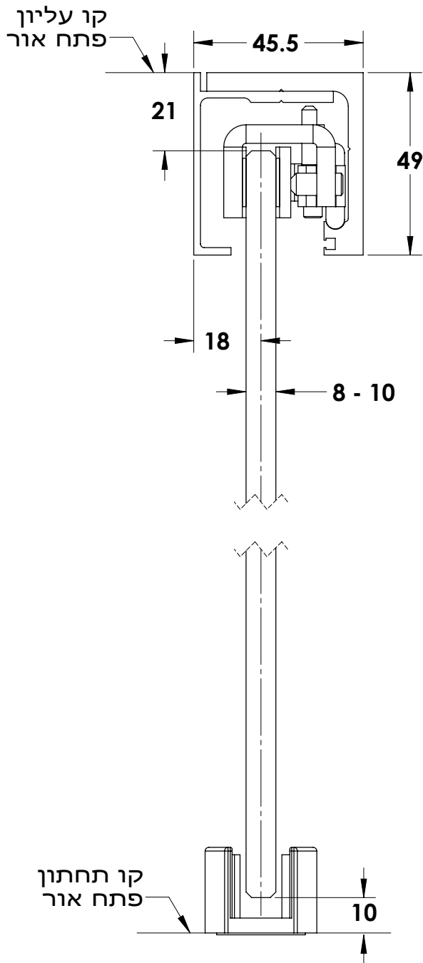
מסילה בחיבור לתיקרה
