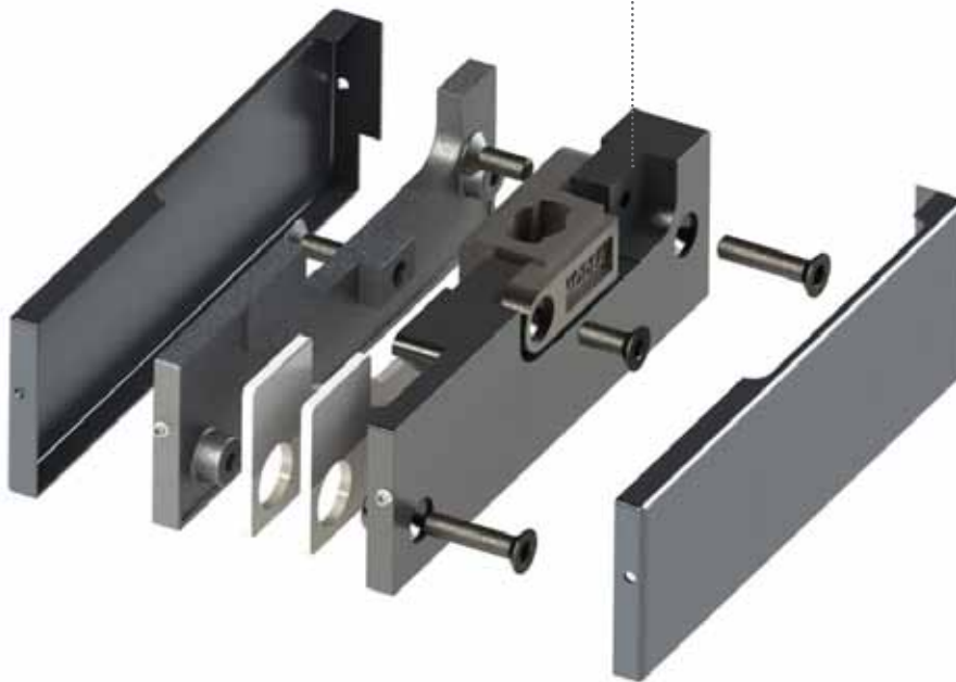
תותב נירוסטה
