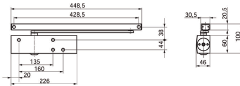
מפרט טכני TS 3000 V
