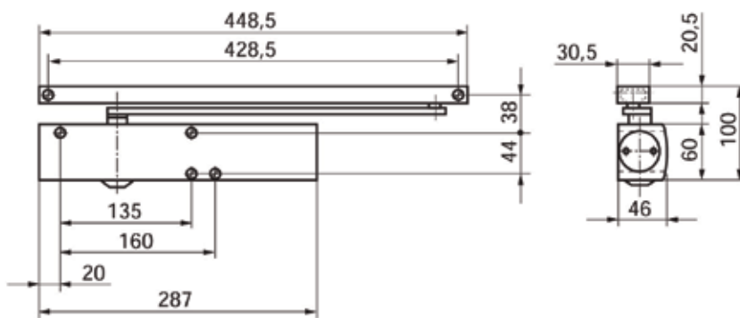
מפרט טכני מחזיר עליון TS 5000 עם זרוע החלקה
