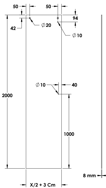
תכנית
