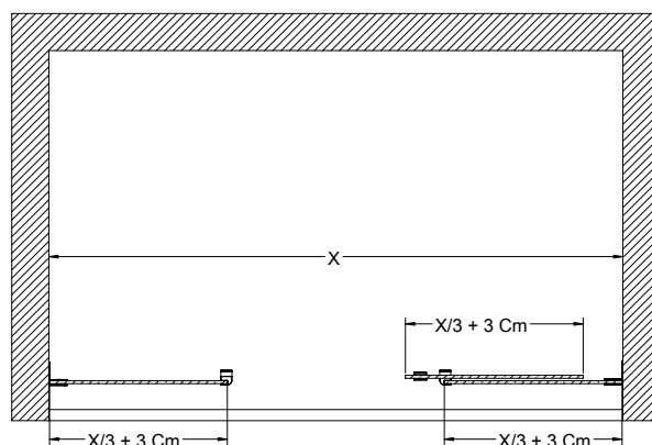
תכנית
